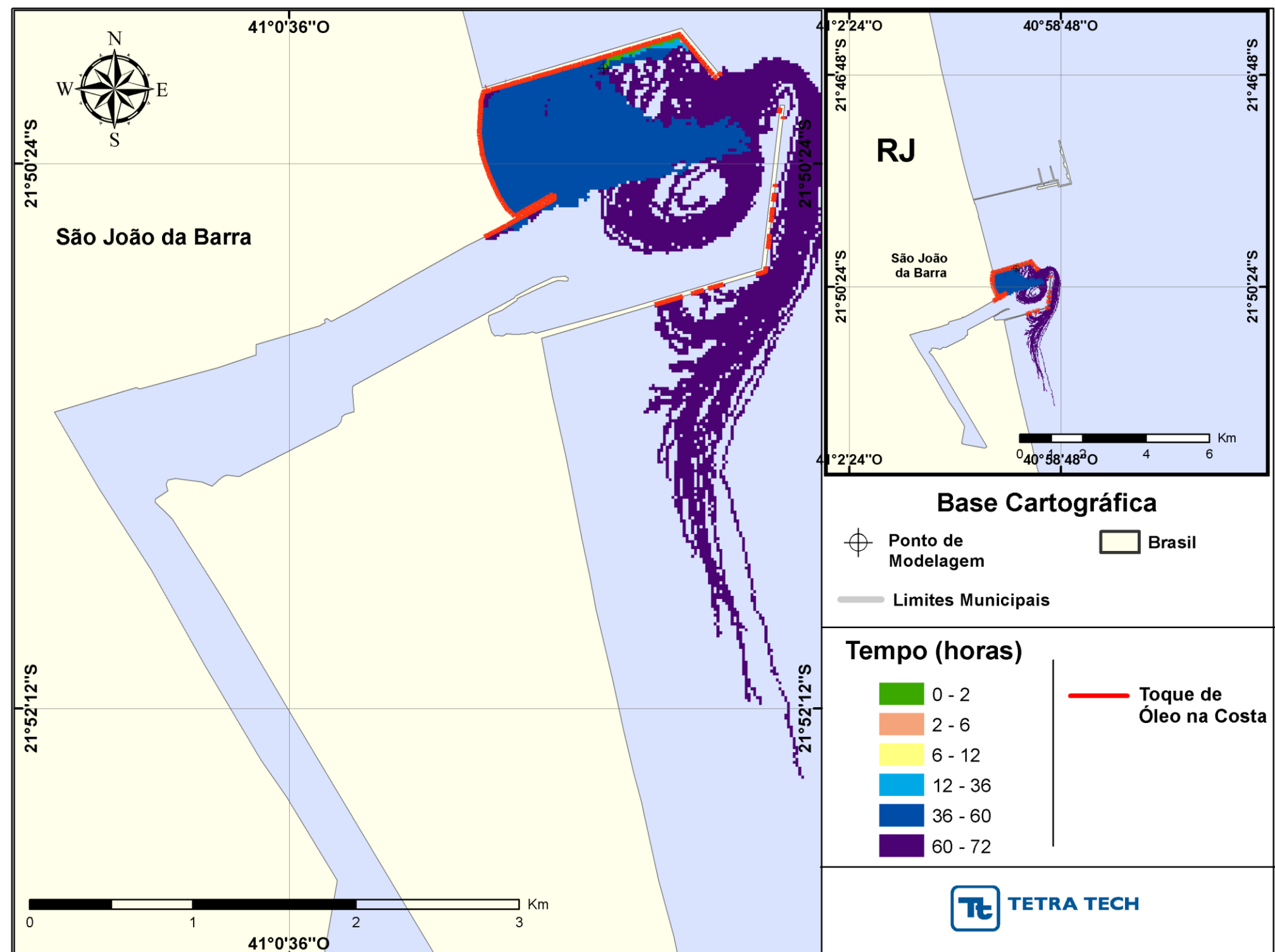
Figura 5.28. Contornos da evolução temporal da mancha de óleo na superfície da água e toque na costa, para a condição de tempo ruim, maré de quadratura, período de vazante, em até 72 horas após o início da simulação, para derramamento de 5.100 m 3 de óleo combustível marítimo MF-380. Datum: SIRGAS 2000.
