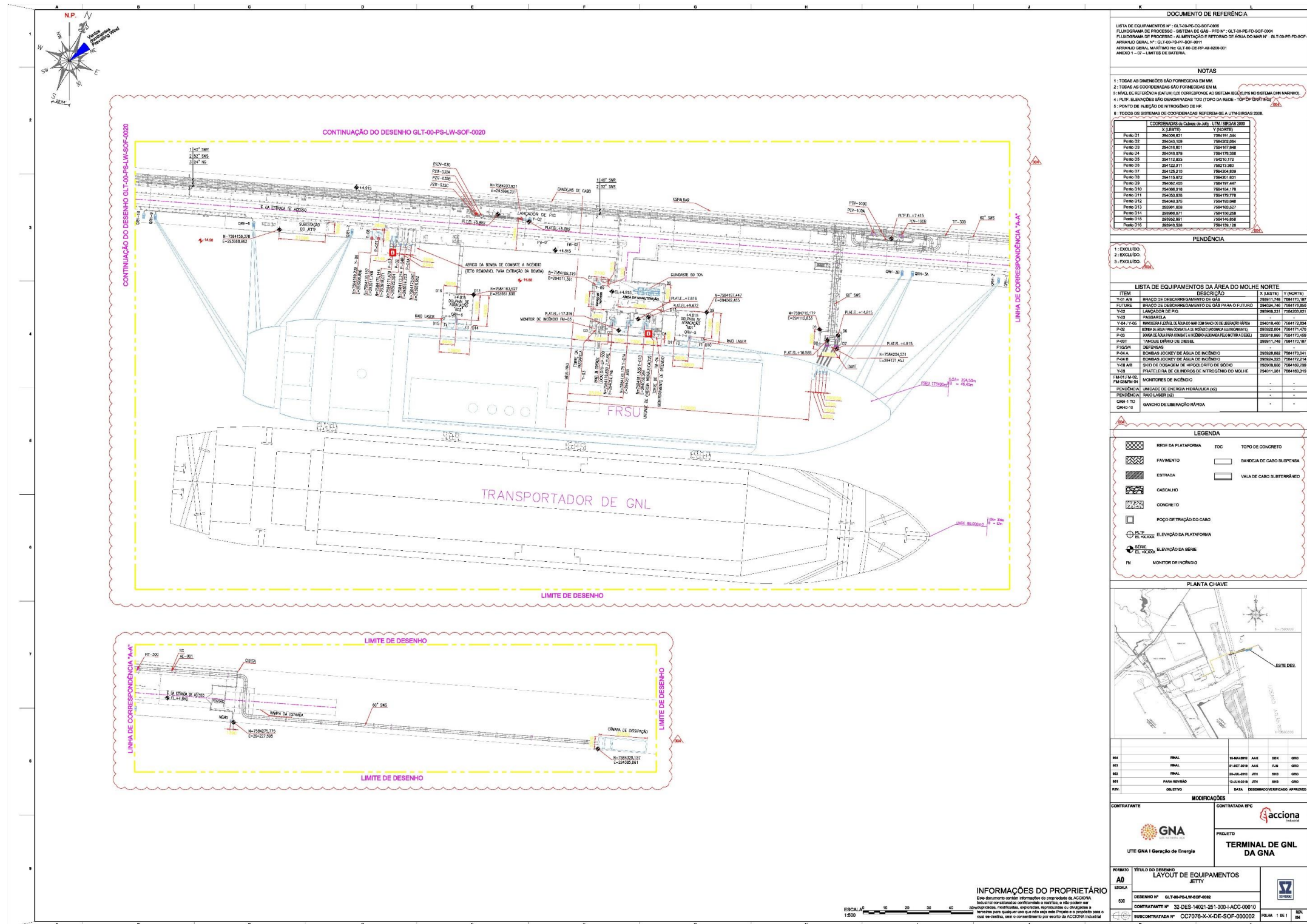
Figura 5.10. Planta da Área do Molhe Norte (atração dos navios - jetty) do TGNL. Datum: SIRGAS 2000.
