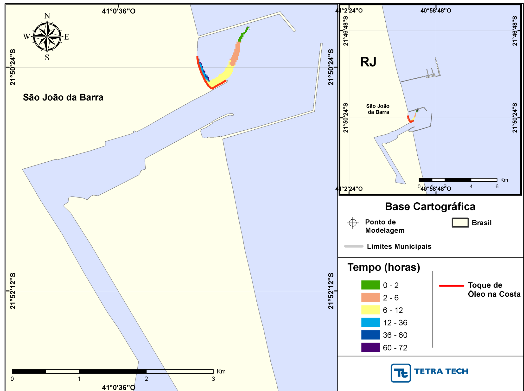
Figura 5.23. Contornos da evolução temporal da mancha de óleo na superfície da água e toque na costa, para a condição de tempo bom, maré de quadradura, período de enchente, em até 72 horas após o início da simulação, para derramamento de 5.100 m 3 de óleo combustível marítimo MF-380. Datum: SIRGAS 2000.
