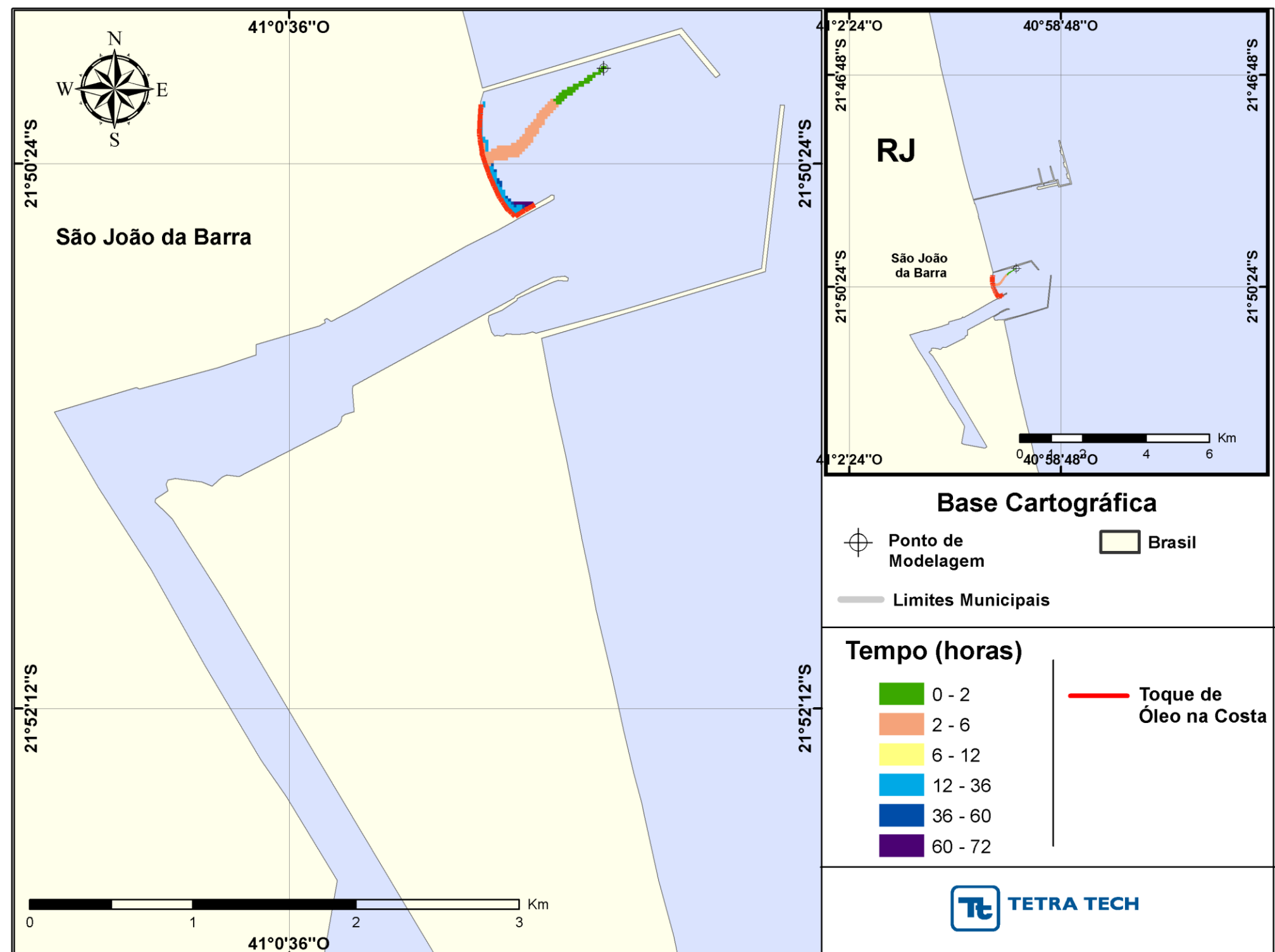
Figura 5.24. Contornos da evolução temporal da mancha de óleo na superfície da água e toque na costa, para a condição de tempo bom, maré de quadratura, período de vazante, em até 72 horas após o início da simulação, para derramamento de 5.100 m 3 de óleo combustível marítimo MF-380. Datum: SIRGAS 2000.
