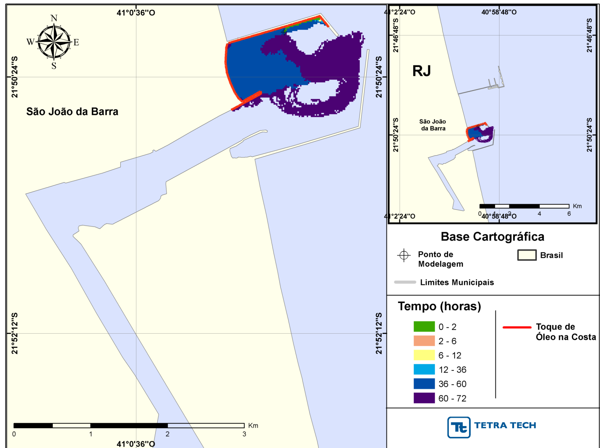
Figura 5.27. Contornos da evolução temporal da mancha de óleo na superfície da água e toque na costa, para a condição de tempo ruim, maré de quadradura, período de enchente, em até 72 horas após o início da simulação, para derramamento de 5.100 m 3 de óleo combustível marítimo MF-380. Datum: SIRGAS 2000.
